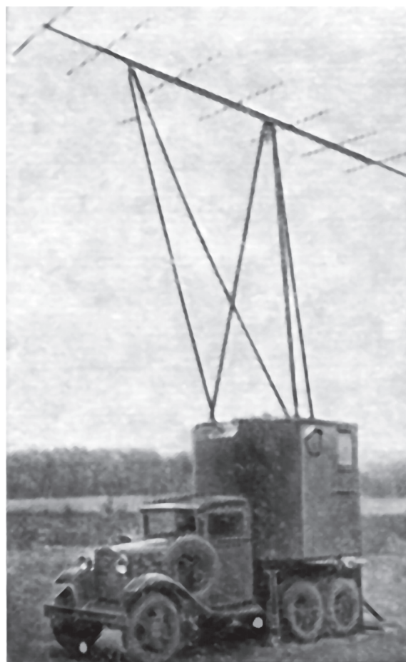
Излучающая установка РЛС РУС-2 («Редут-40») на шасси автомобиля ГАЗ-ААА.
