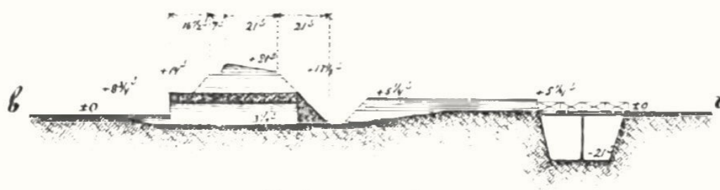
Профиль по линіи в г.
