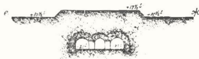
Профиль по линіи е ж.
